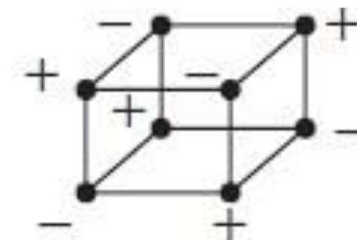
Octopole ( V \sim 1/r^4 )
