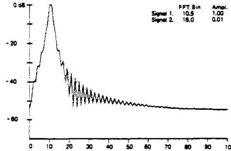
Fig. 79. Poisson window ( \alpha = 3.0 ).
