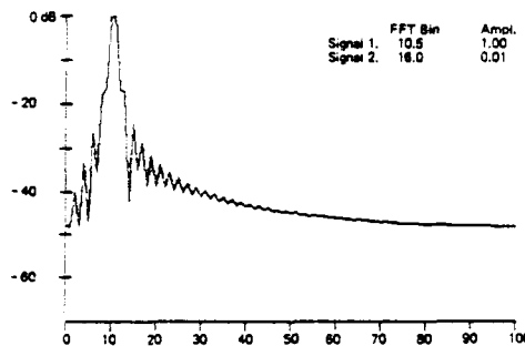
Fig. 78. Poisson window ( \alpha = 2.0 ).
